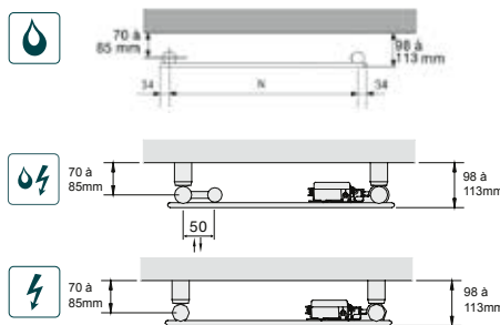
Cotes de perçage
