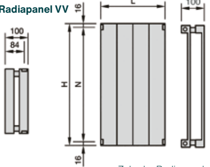
Zehnder Radiapanel anciennement nommé Panneau 87
