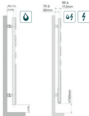
Saillie au mur
