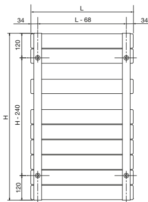
Cotes de perçage
