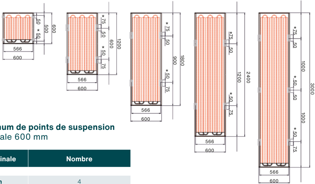
Schémas indiqués en largeur standard et 6 tubes. Existe aussi en version 4 tubes, pour un encombrement identique.
